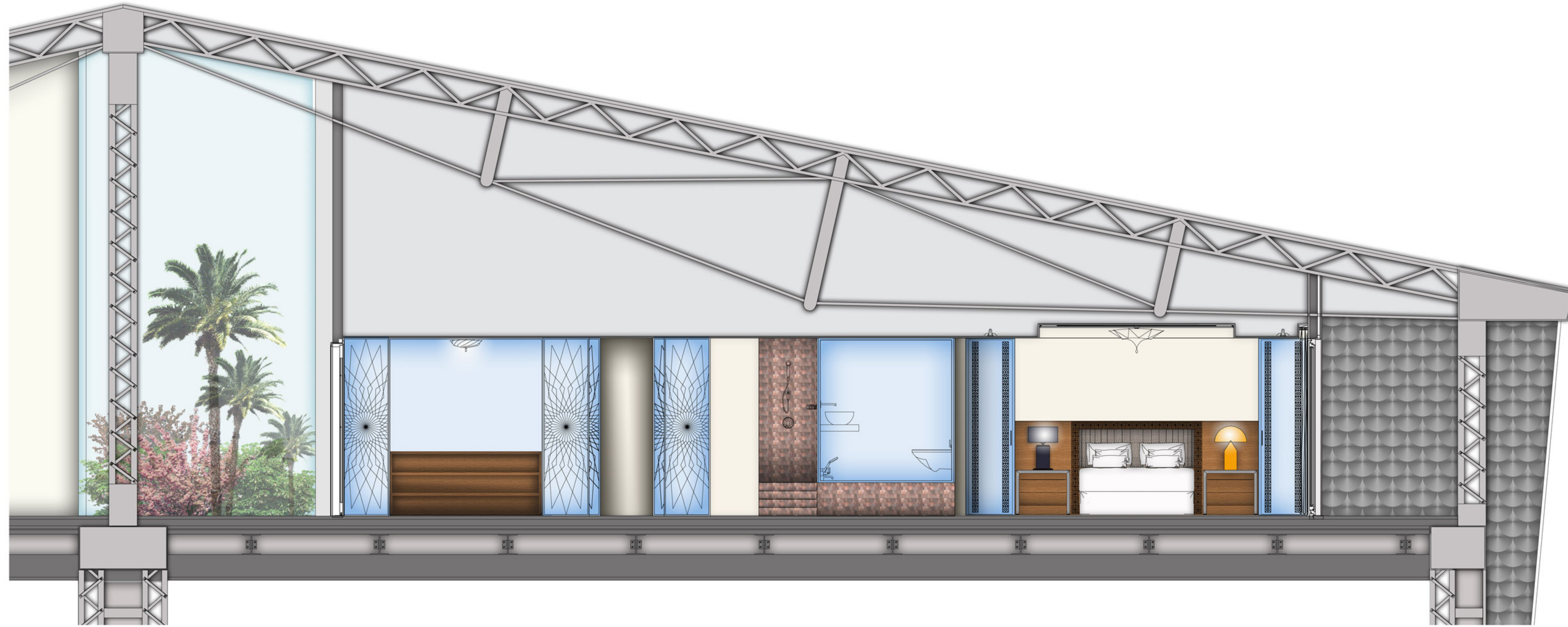
Sezione King Suite Scala 1:50
