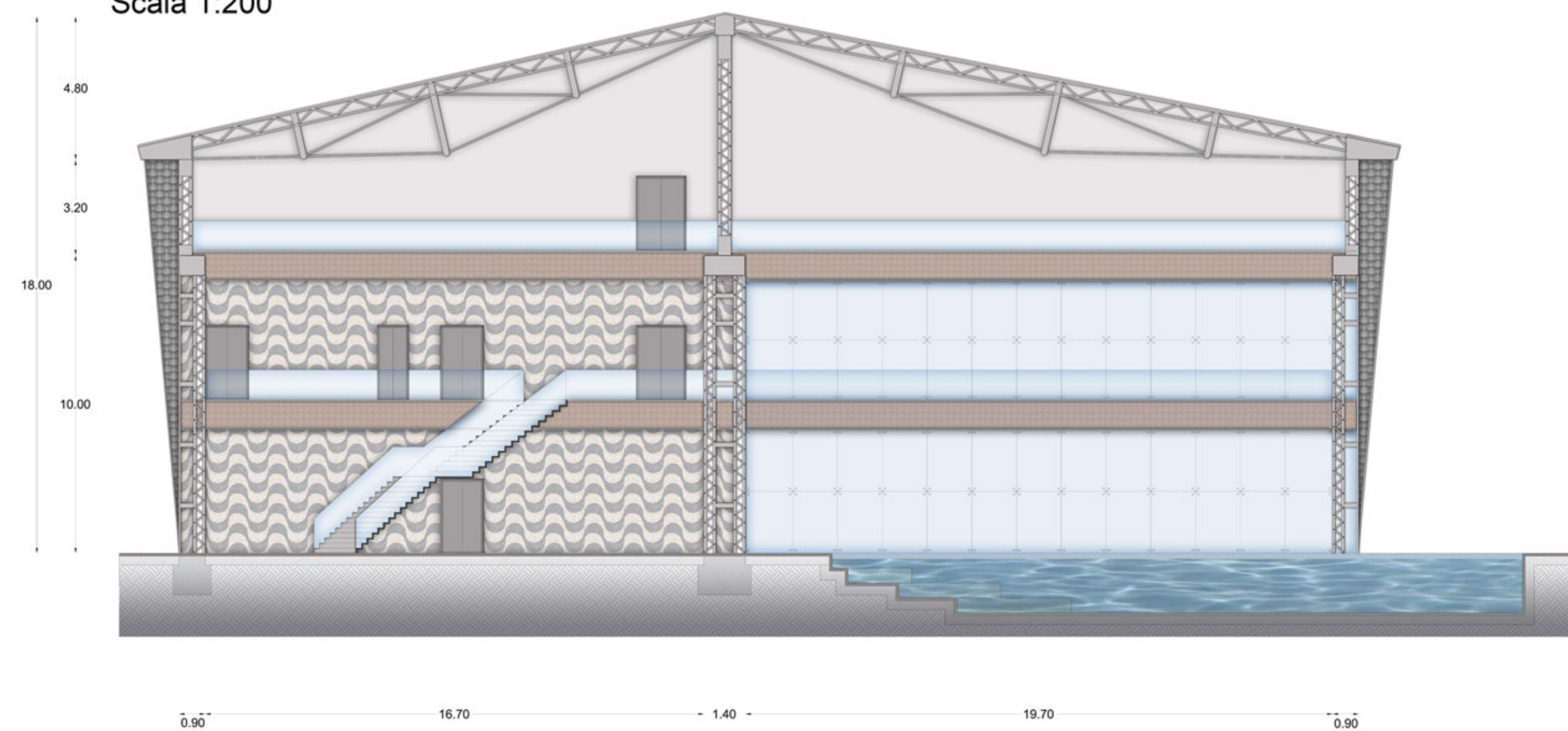
Sezione C-C Scala 1:200
