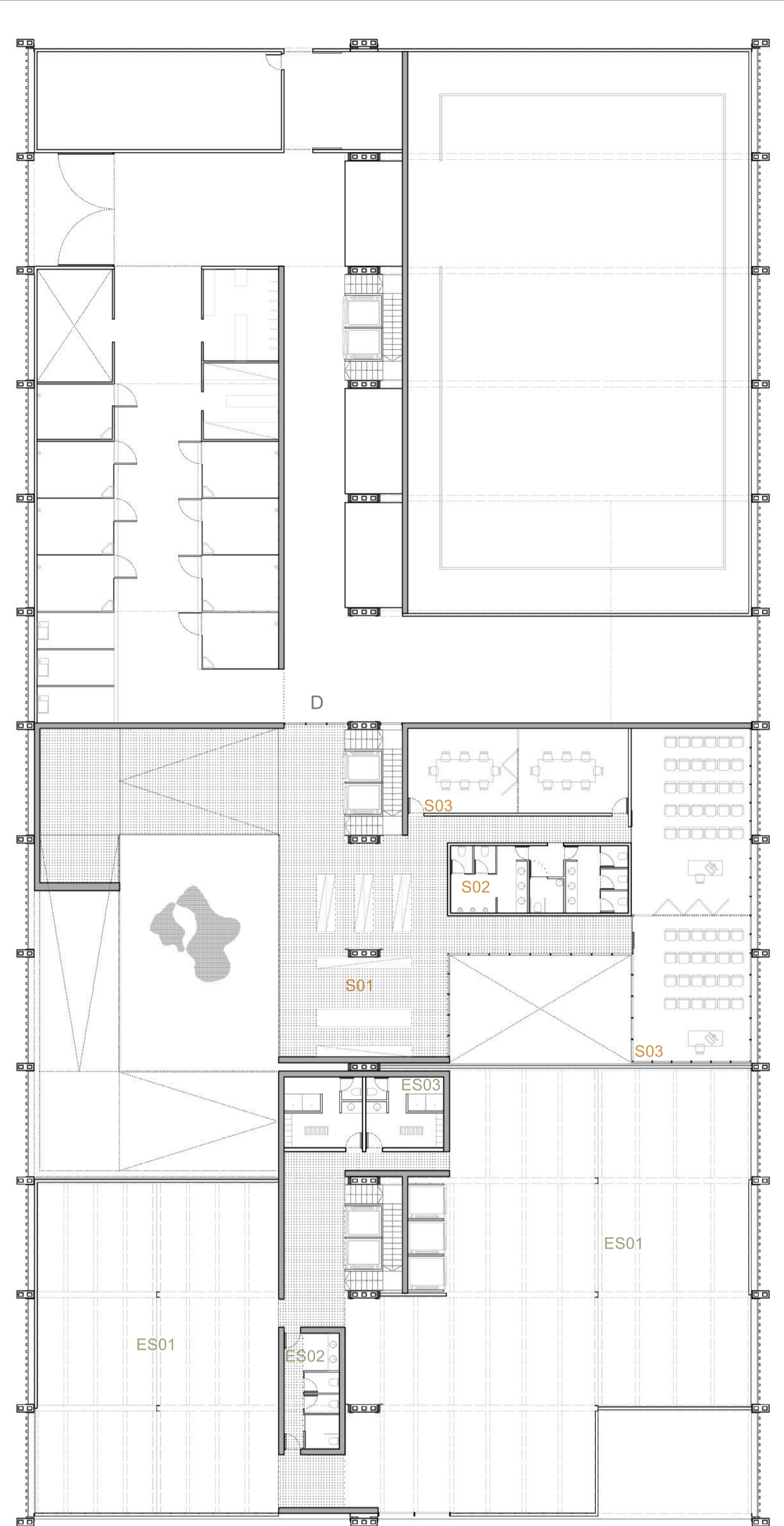
PIANTA 3.65
